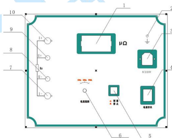
图一 面板布局图
