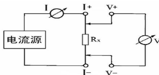
图二 测试原理图
